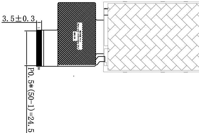
背视图
