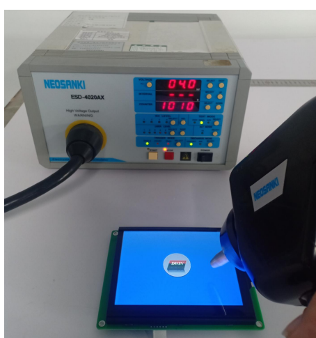
3.1 静电放电测试图
