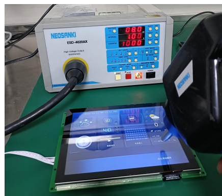
3.1 静电放电测试图
