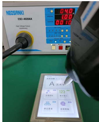
3.1 静电放电测试图
